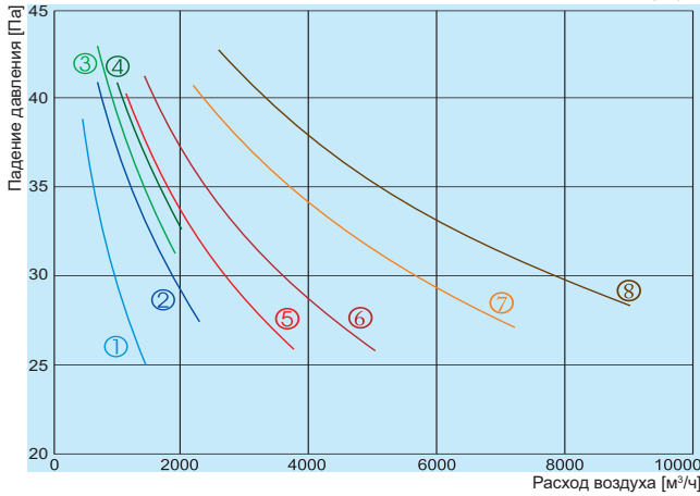
Повышение температуры при объеме потока воздуха, воды 80 ° / 60 °C \rho = 1.20 \text{ кг/м}^3
